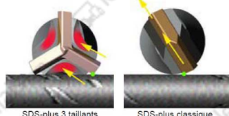
SDS-plus 3 taillants
