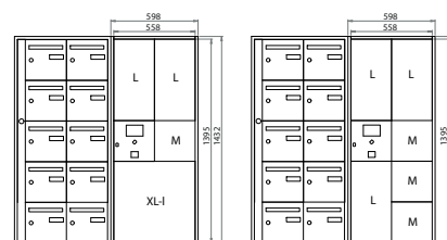
Exemples d'intégration MyColisBox avec un bloc collectif d'une hauteur de 5 cases
