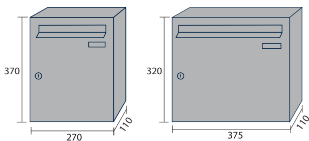
Dimensions extérieures d'une boîte
