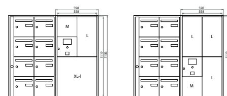
Exemples d'intégration MyColisBox avec un bloc collectif d'une hauteur de 4 cases
