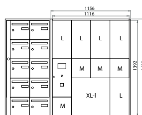
Exemple d'intégration MyColisBox avec un bloc collectif d'une hauteur de 5 cases
