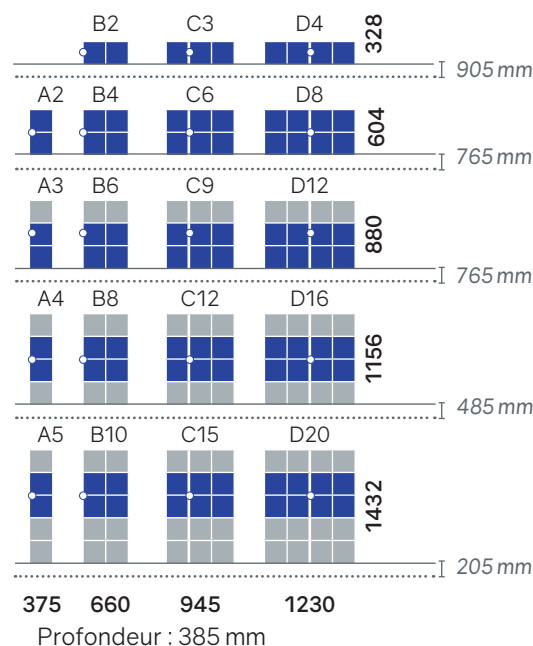
Dimensions intérieures d'une boîte
