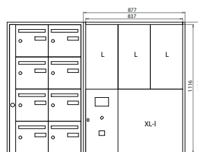
Exemple d'intégration MyColisBox avec un bloc collectif d'une hauteur de 4 cases
