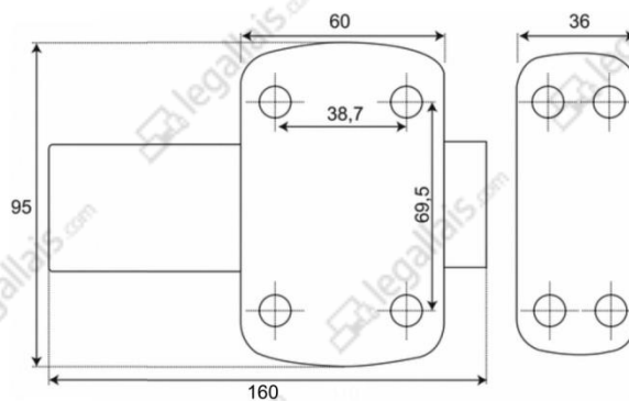
Pêne rallongé
