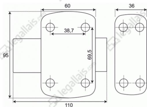
Pêne standard
